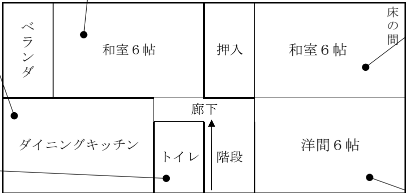
2階
